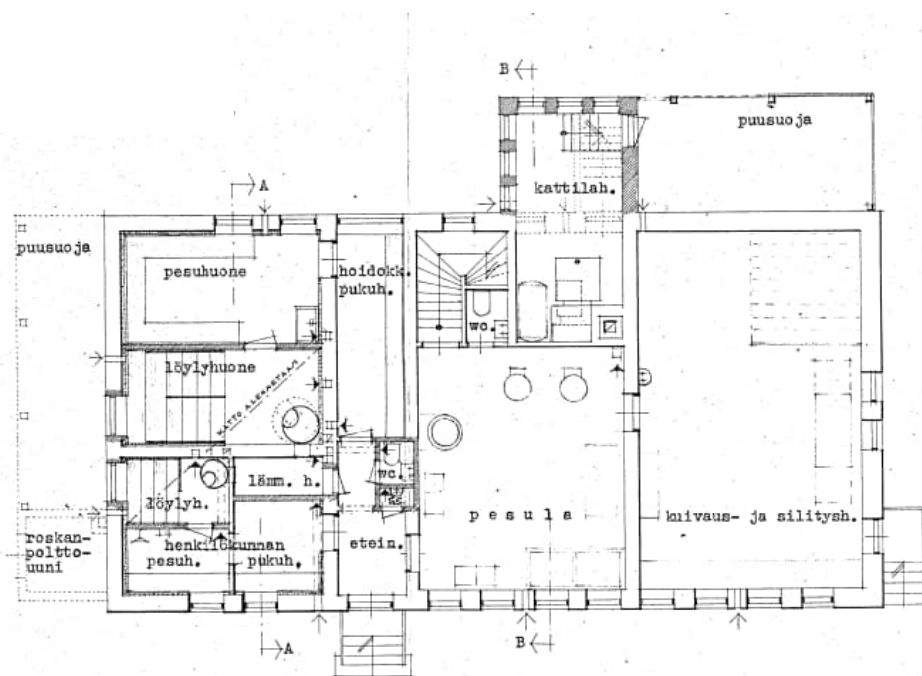
Kuva 2. Hyväksytty pohjakuva vuoden 1959 tehdyistä muutoksista. Muutostyöt suunnitellut arkkitehti Olaf Kuttner vuonna 1958. (Kuva saatu Porin kaupungin rakennusvalvontayksiköstä).
