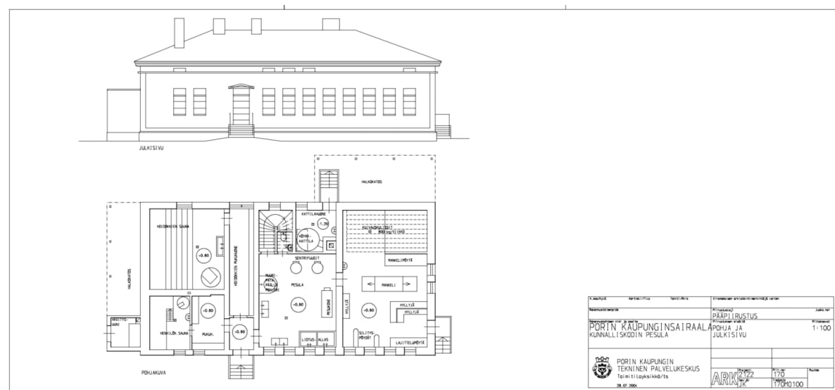
Pääpiirustus, 1:100, pohja ja julkisivu
