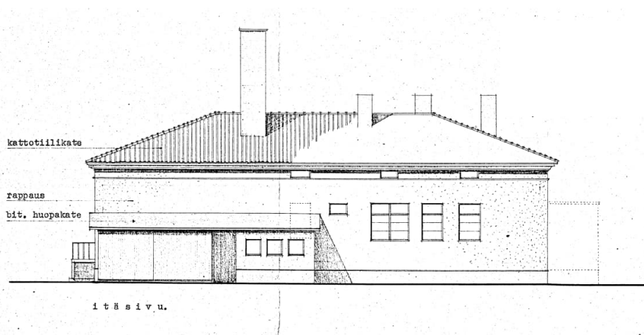
Kuva 5. Hyväksytty julkisivu kuva vuoden 1959 tehdyistä muutoksista. Muutostyöt suunnitellut arkkitehti Olaf Kuttner vuonna 1958. (Kuva saatu Porin kaupungin rakennusvalvontayksiköstä).
