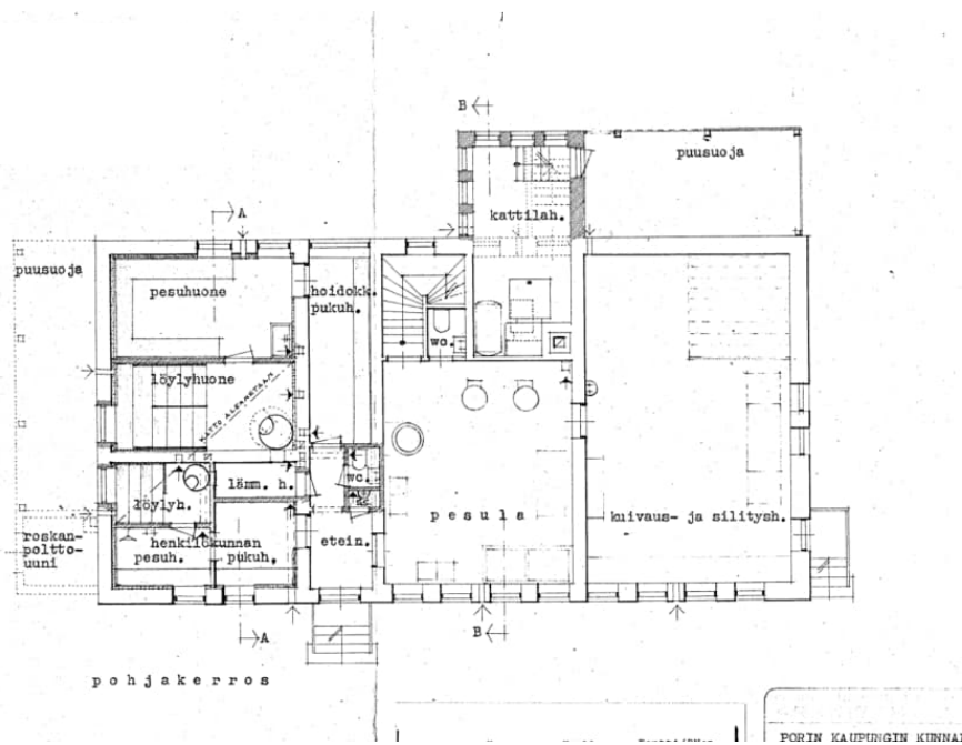
Kuva 19. Rakennuksen pohjakuva vuonna 1959 tehdyn laajennuksen jälkeen.
